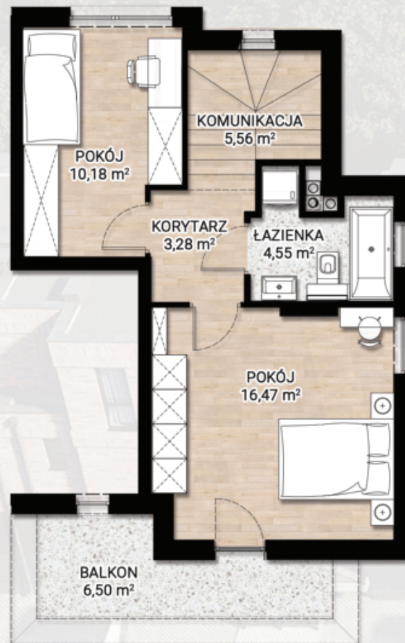
RZUT PIĘTRA I
