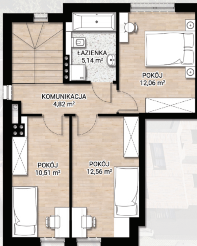
RZUT PIĘTRA I
