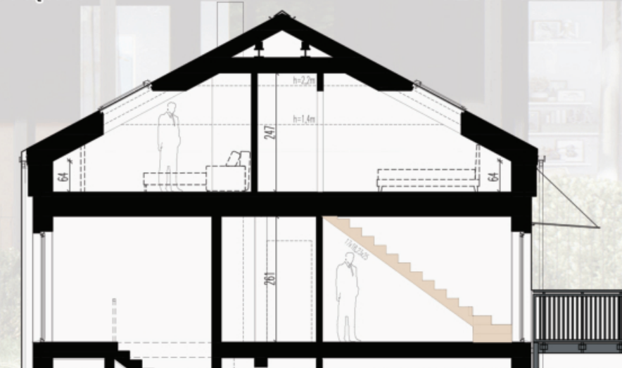
PRZEKRÓJ
