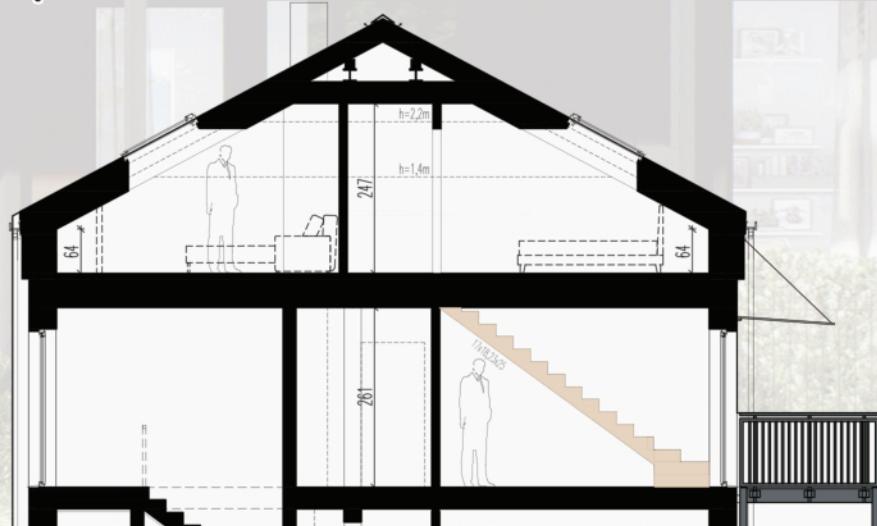
PRZEKRÓJ
