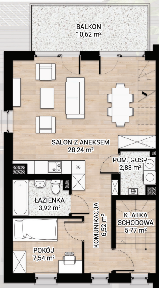
RZUT PIĘTRA
